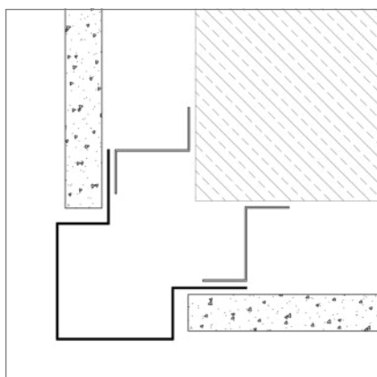
vnější roh
