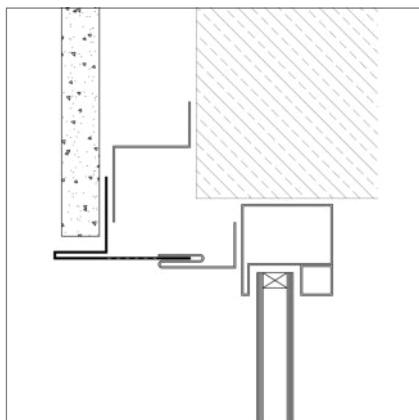
okenní překlad varianta 1
