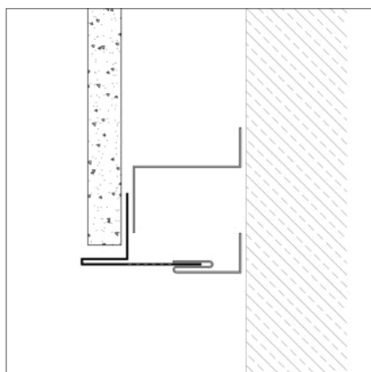
ukončení soklu
