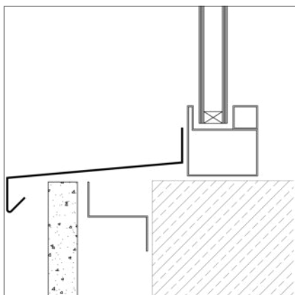
okenní parapet
