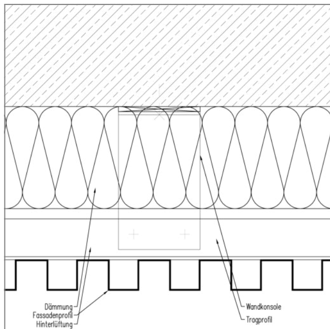
Skladba fasády: Horizontální řez s meandrovitým profilem
