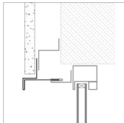
okenní překlad varianta 2
