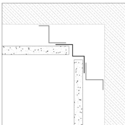
vnitřní roh
