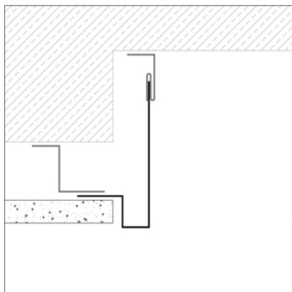
okenní ostěň
