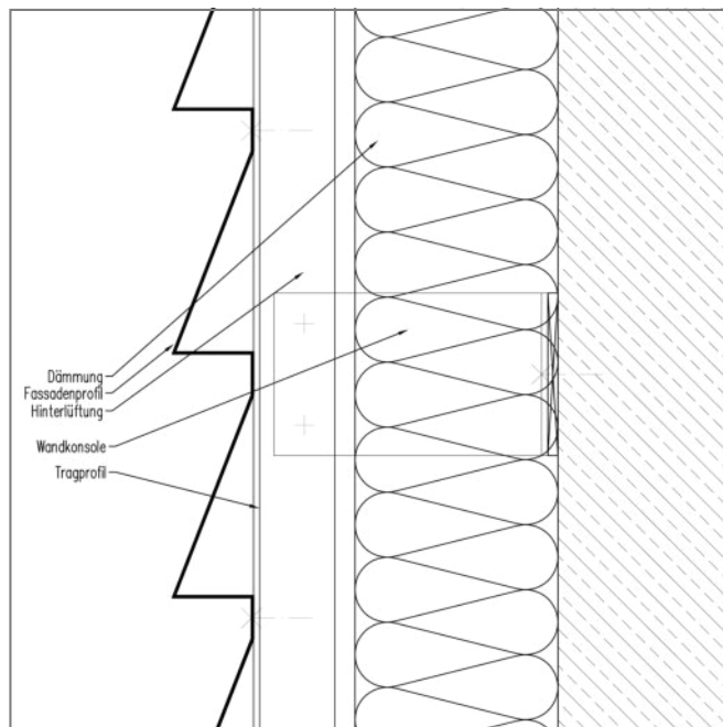
Skladba fasády: Vertikální řez s pilovitým profilem
