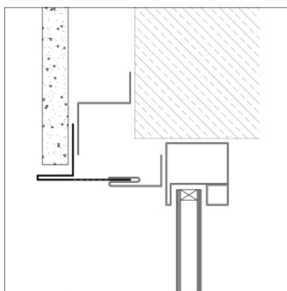
okenní překlád varianta 1
