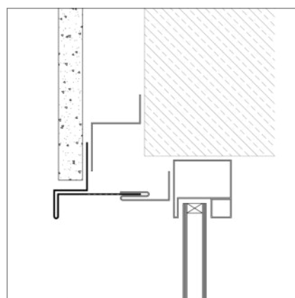
okenní překlád varianta 2
