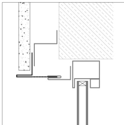
Fenstersturz Variante 1
