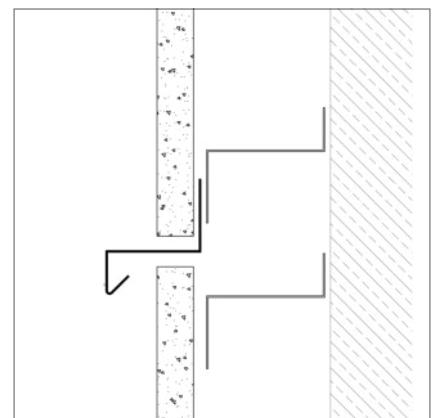
Querstoss
