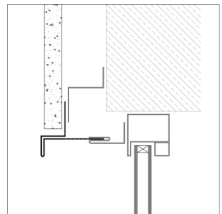
Fenstersturz Variante 2
