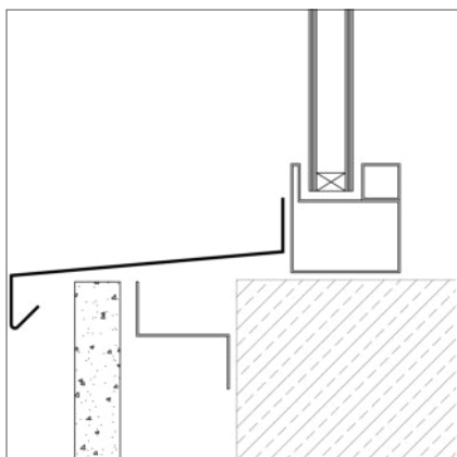
Parapetová doska
