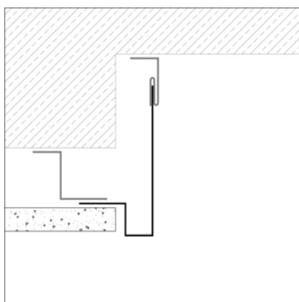
Okenné ostenie
