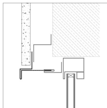
Okenný preklad variant 2
