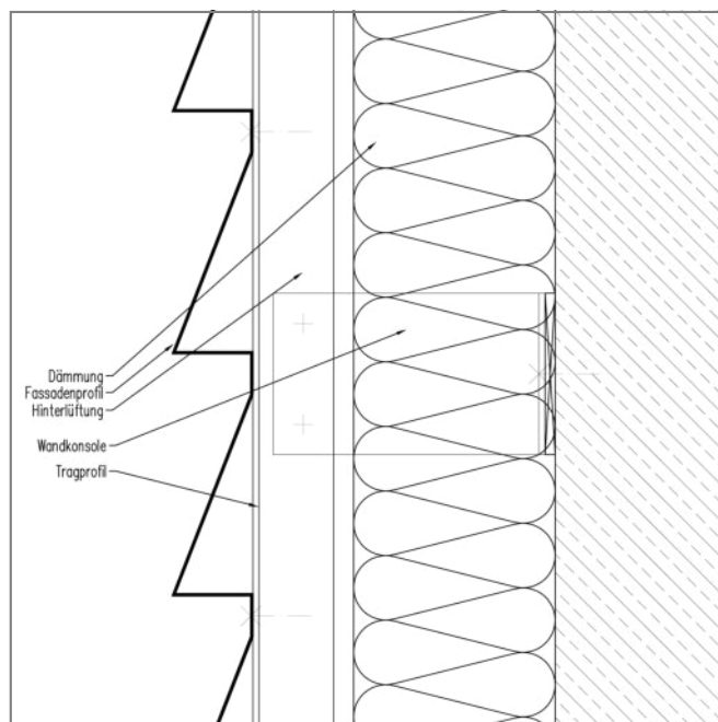
Zloženie fasády: Vertikálny rez s pílovým profilom
