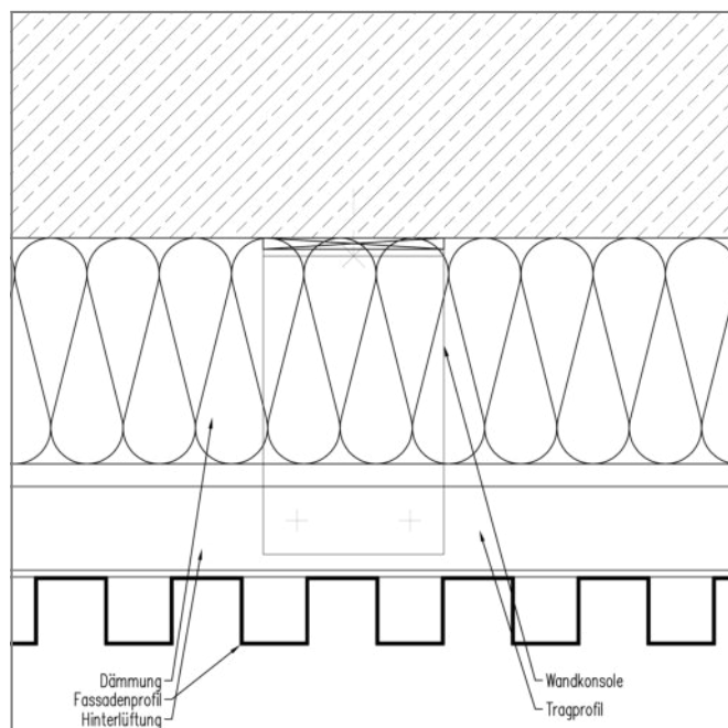
Zloženie fasády: Horizontálny rez s meandrovitým profilom
