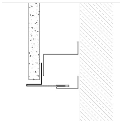
Soklová koncovka
