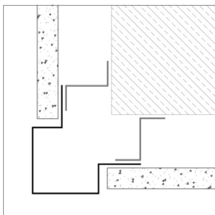
Vonkajší roh
