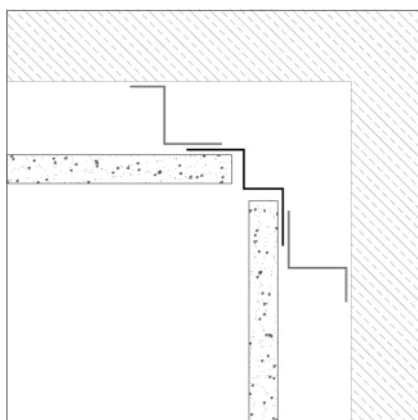
Vnútorňý roh
